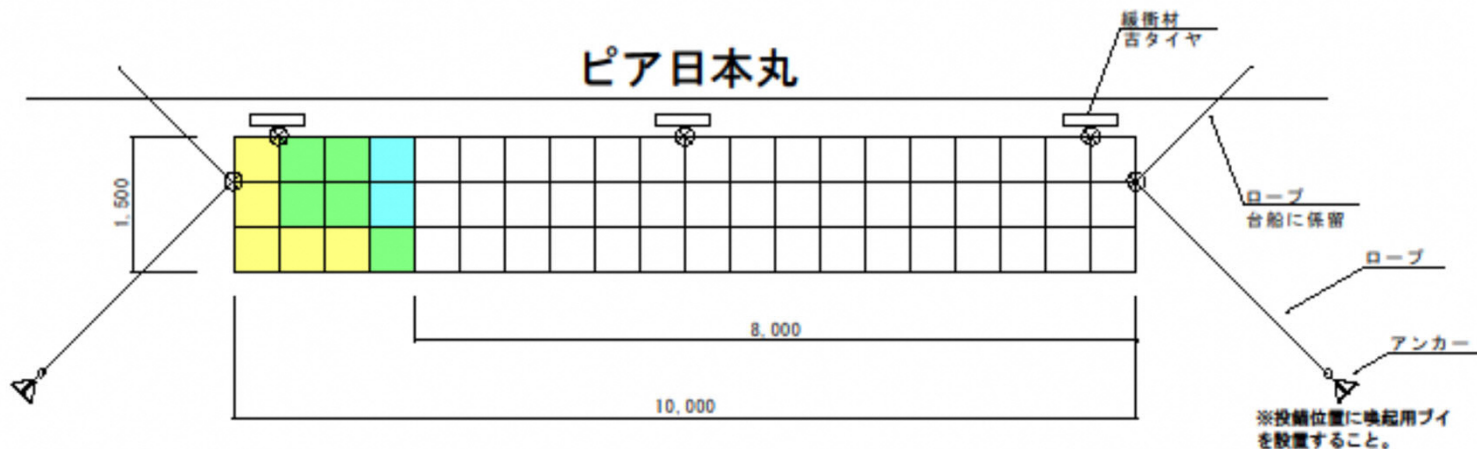
平面図
