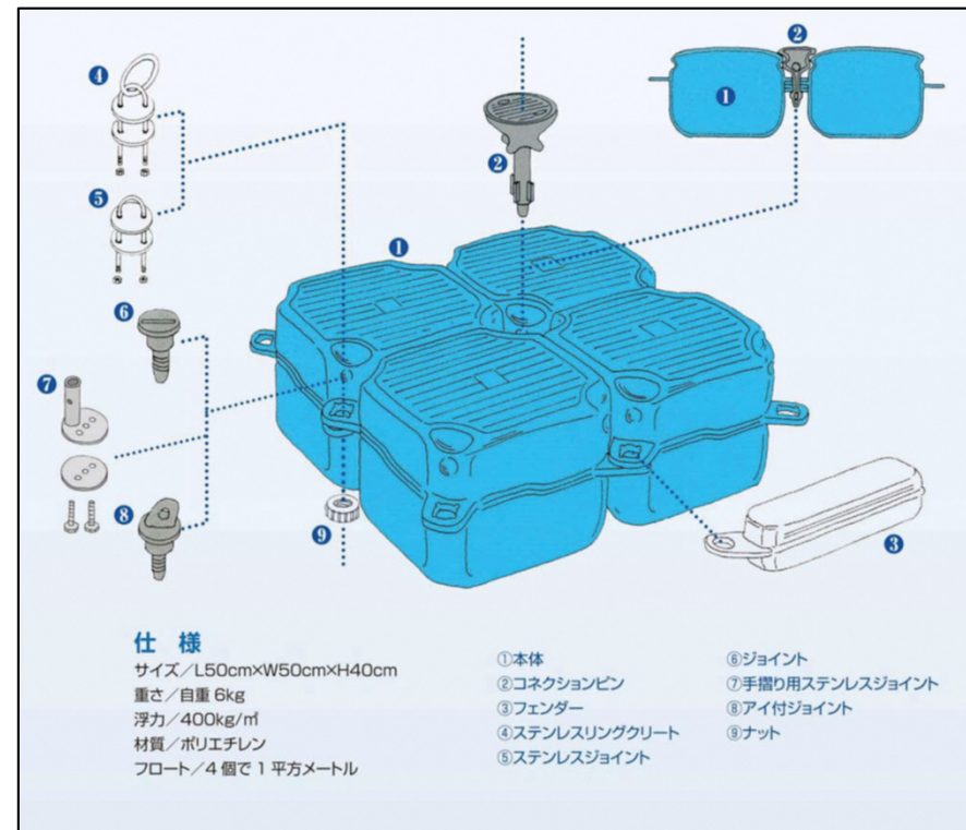
<参考>ピアフロート仕様図
