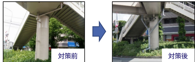
＜歩道橋の耐震化事例＞
