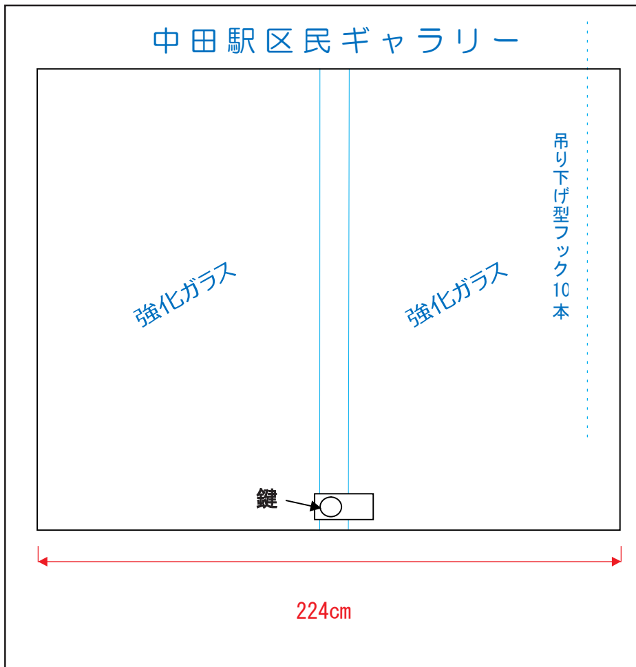
(正面寸法)
