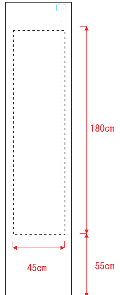
(側面寸法)
