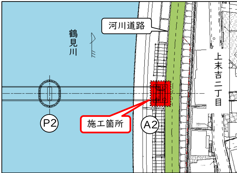
鋼矢板圧入
