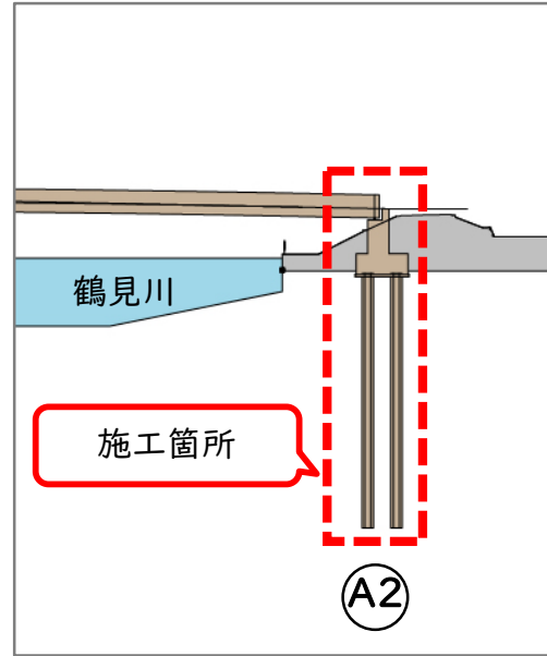
鋼矢板圧入
