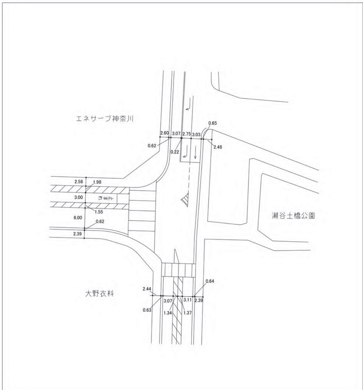
図 9.17-4(6) 交差点構造図 (地域社会 4 : 瀬谷土橋公園前交差点)
