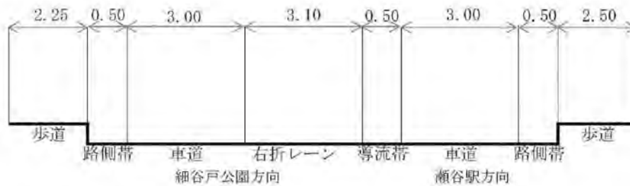
図 9.17-3(3) 道路構造図 (地域社会 7)
