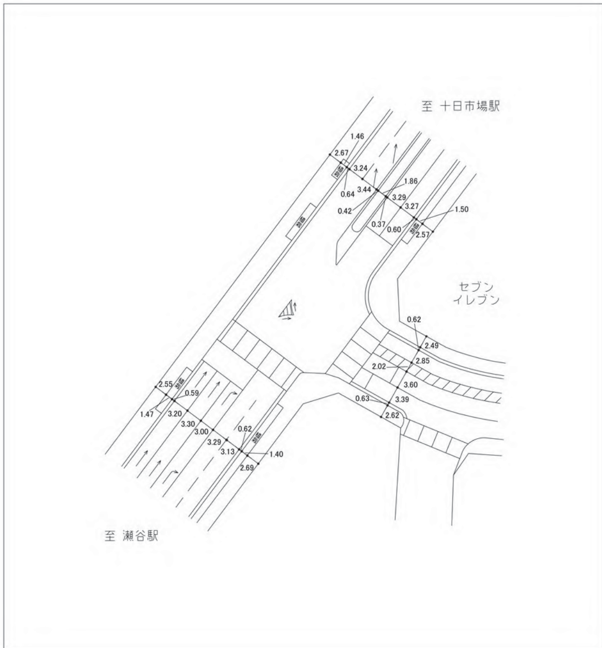
図 9.17-4(5) 交差点構造図 (地域社会 4 : 瀬谷土橋公園入口交差点)
