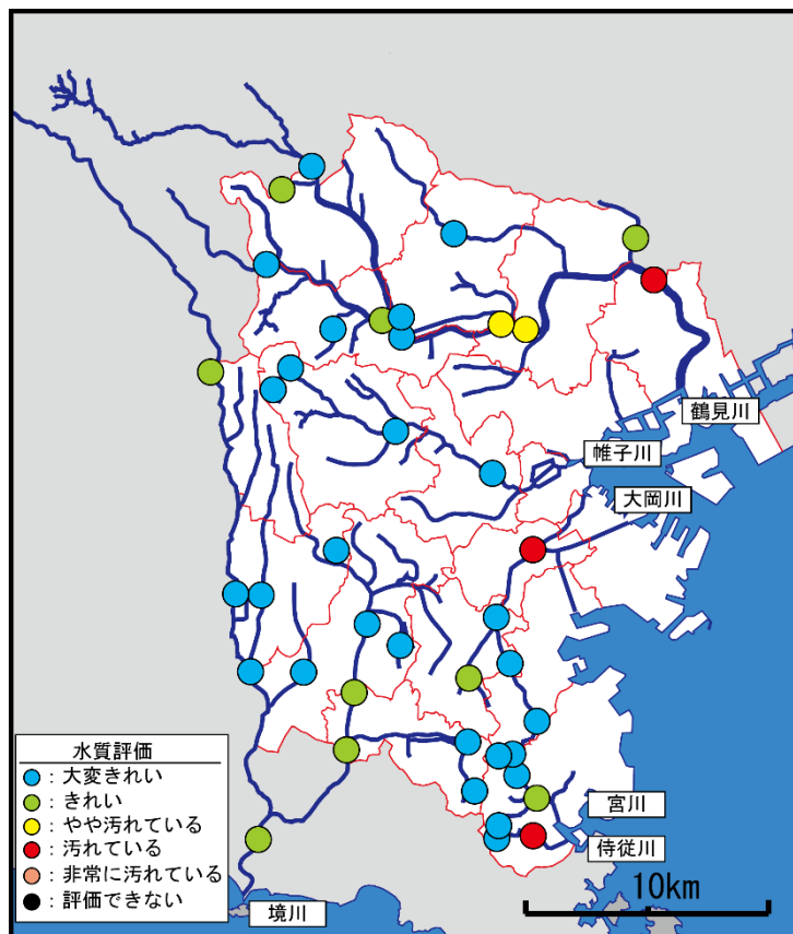
図3 横浜市内河川の水生生物による水質評価結果（2019年度夏季）
