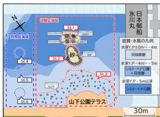
図2 平面図
