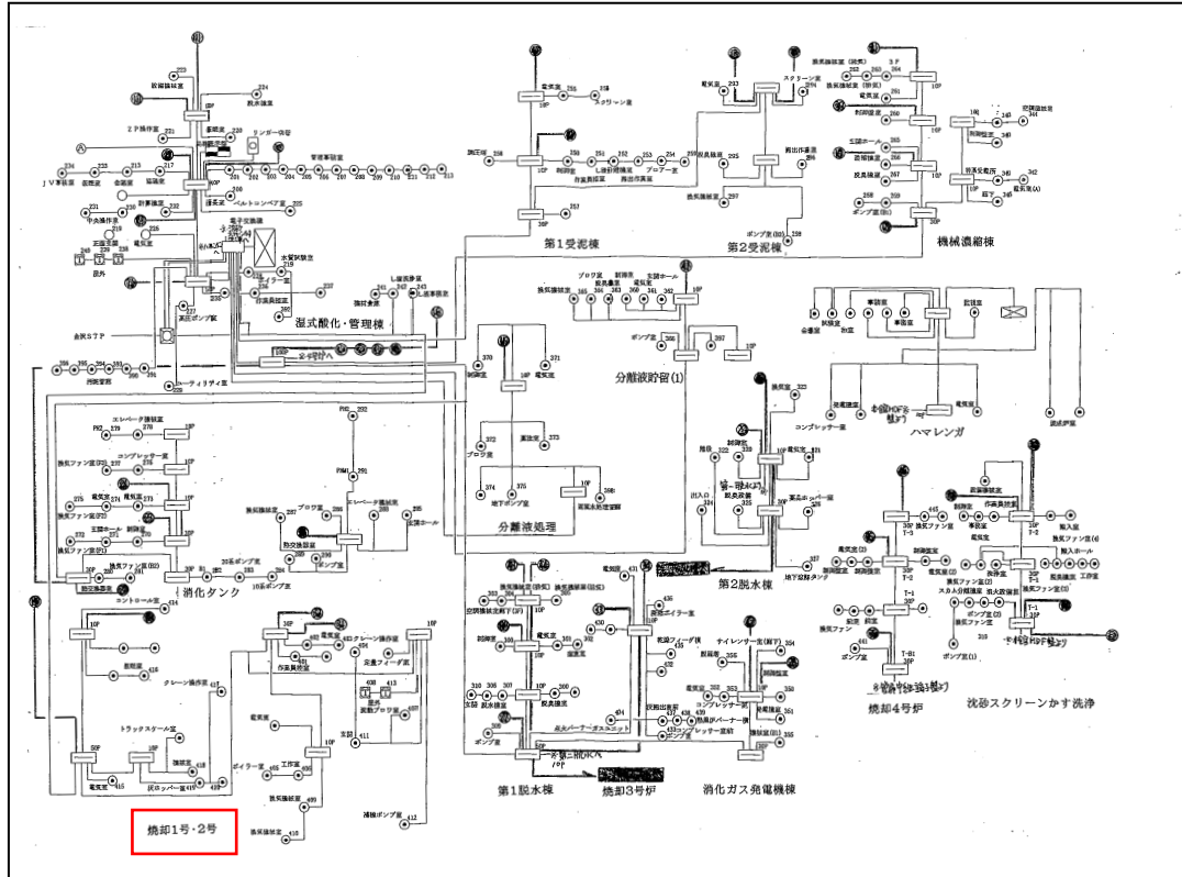
電話系統図 (赤枠が該当箇所)
