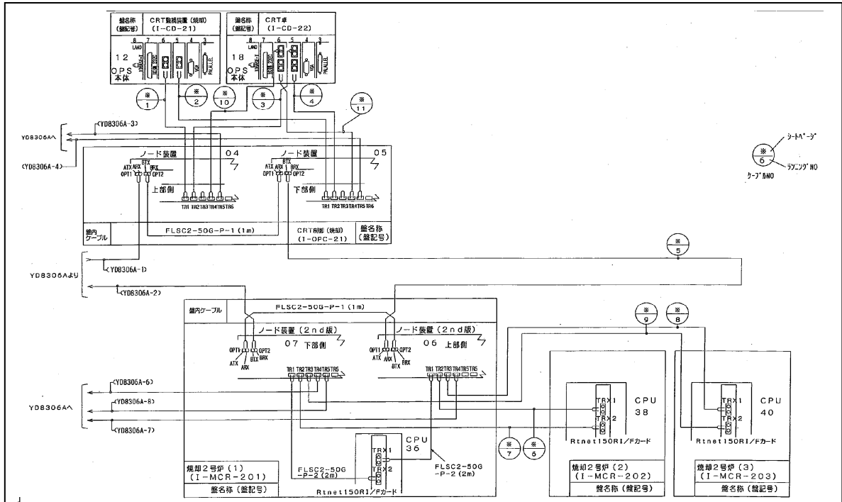
既設汚泥焼却炉2号炉 監視システム構成図
