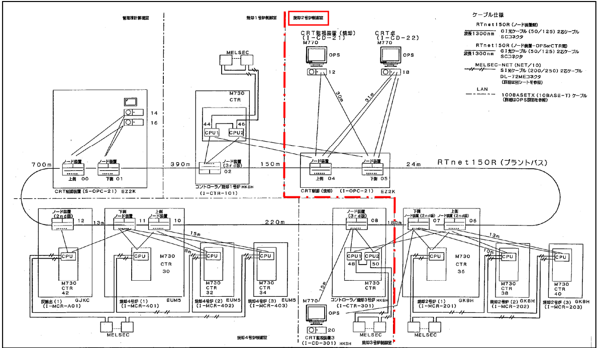
南部汚泥資源化センター監視システム構成図
