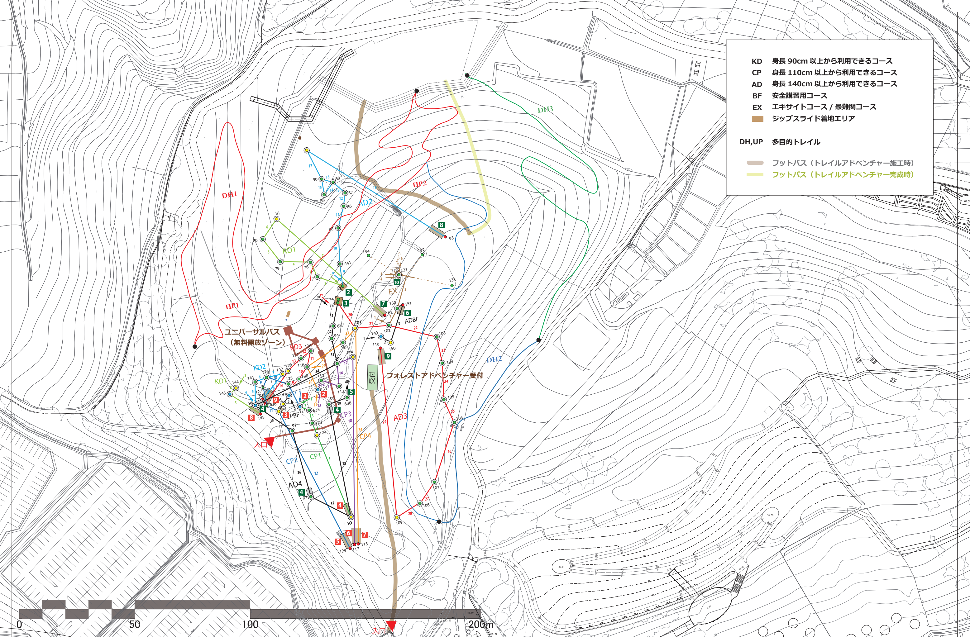
全体レイアウト図
