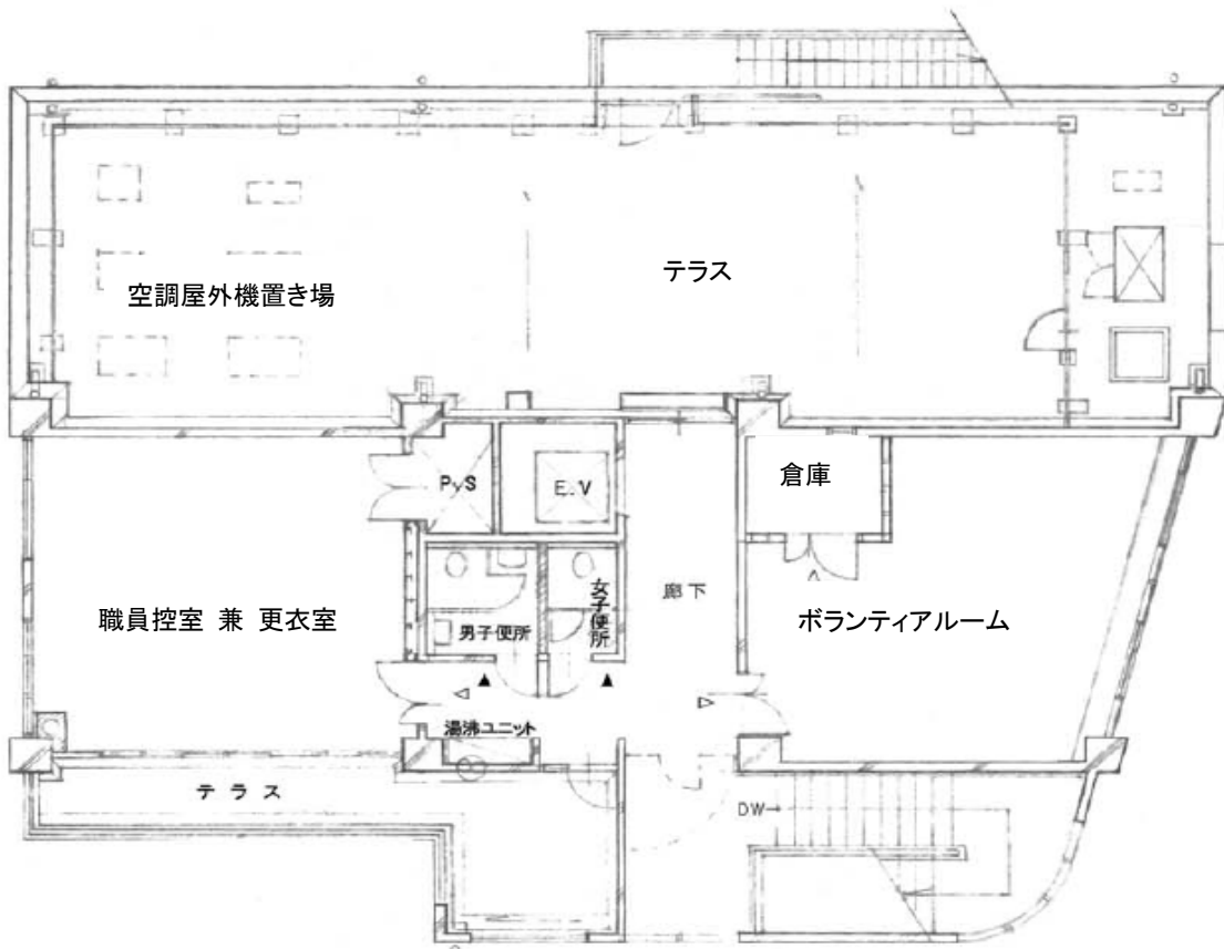
3階 竣工図
