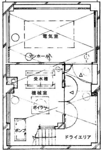
地階竣工図
