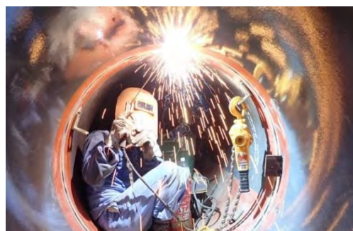
老朽管耐震更新工事（管内溶接）
