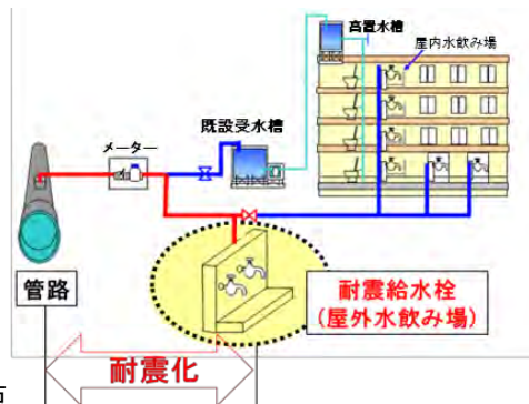
耐震給水栓の概要
